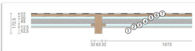
Figuur 8: H02 Hellend dak (45°) met ALU Seal 45 onder het dakbeschoot tussen de balkconstructie
