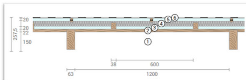
Figuur 7: H01 Hellend dak (45°) met ALU Seal 45 op het dakbeschoot
